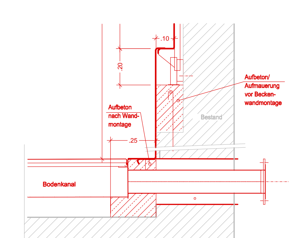
Detail A o. M. Schwimmer- und Springerbecken (SSB) Bodenkanaleinspeisung
