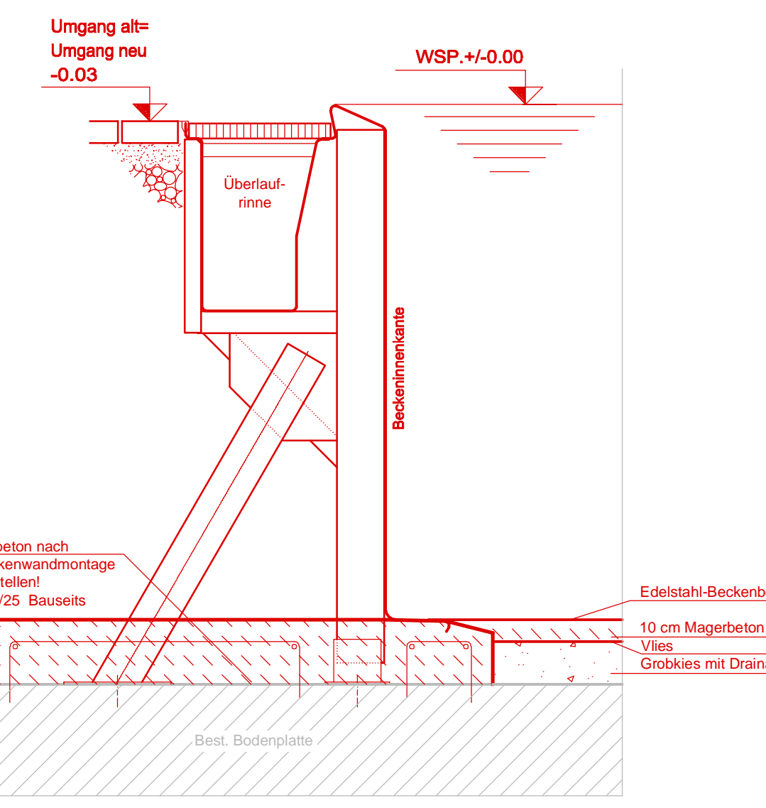
Detail C o. M. Überlaufrinne (neuer Beckenrand)
