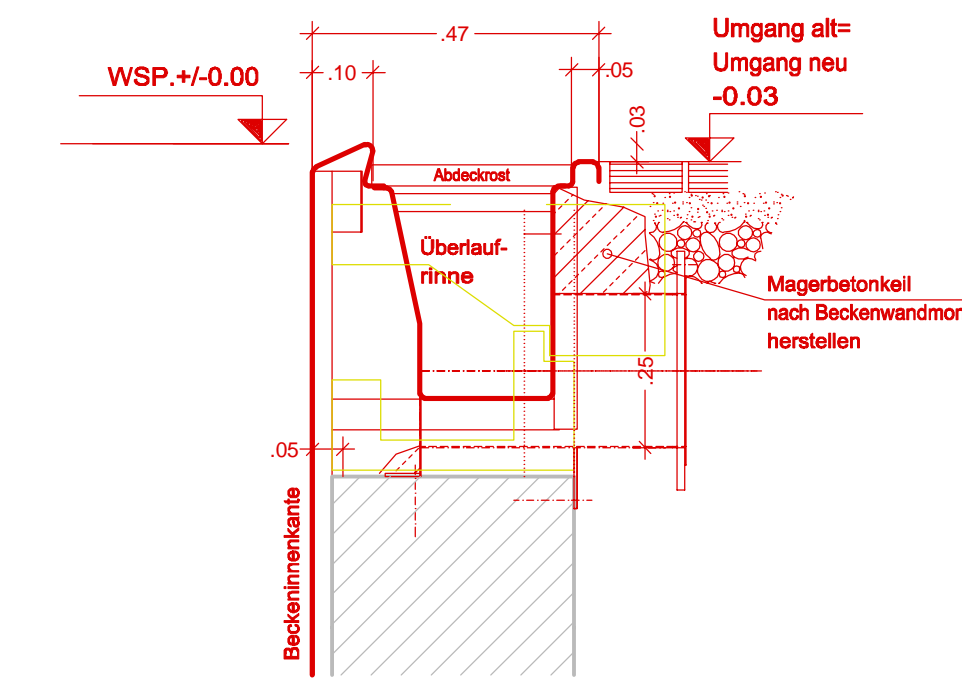
Detail B o. M. Schwimmer- und Springerbecken (SSB) Überlaufinnenablauf
