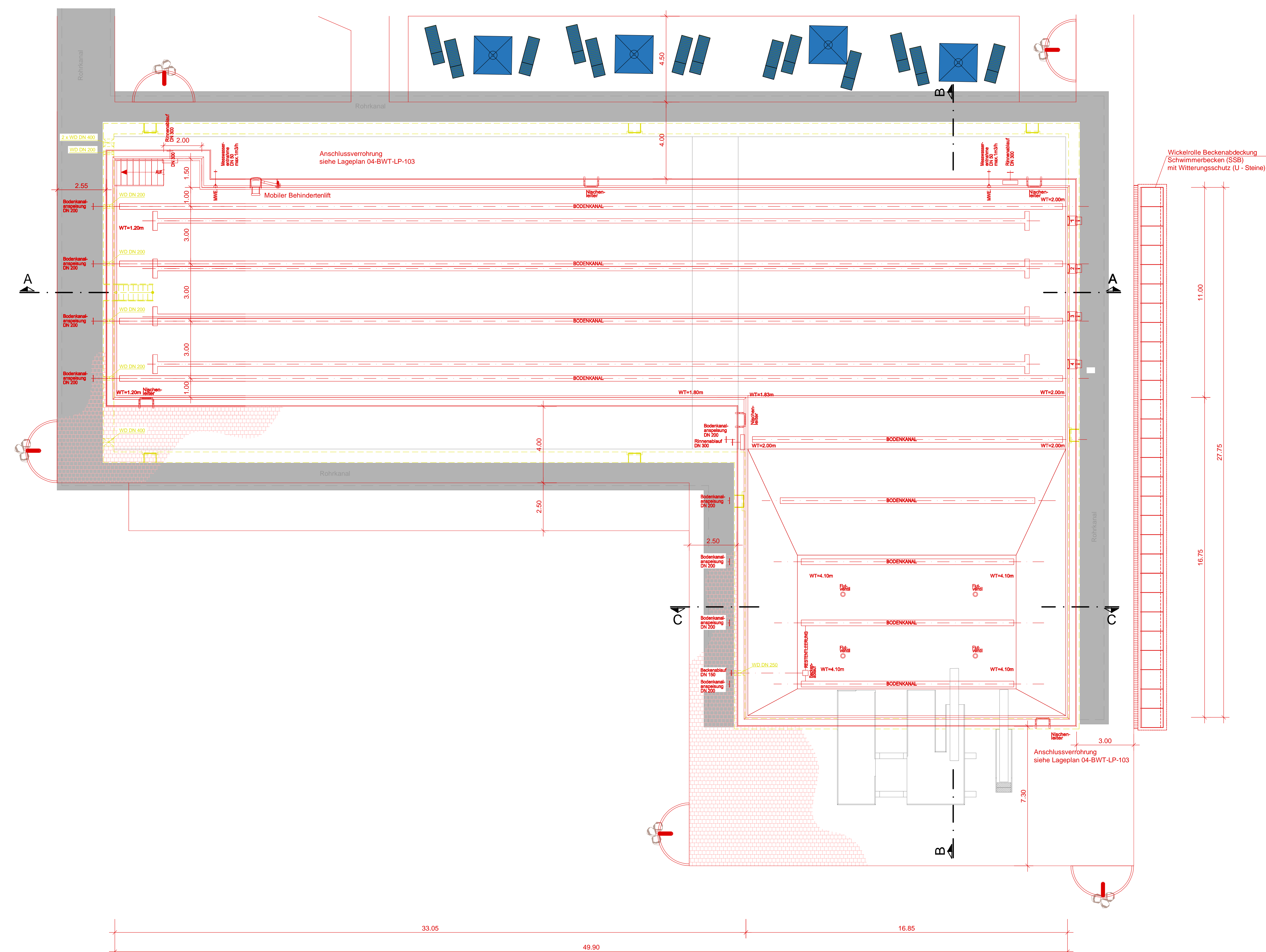
Detail A o. M. Schwimmer- und Springerbecken (SSB) Bodenkanaleinspeisung
